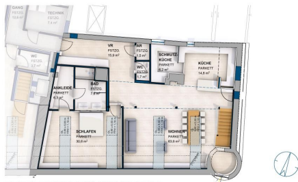
PENTHOUSE 2 (INKL. FLÄCHE <150cm) - M 1:100
